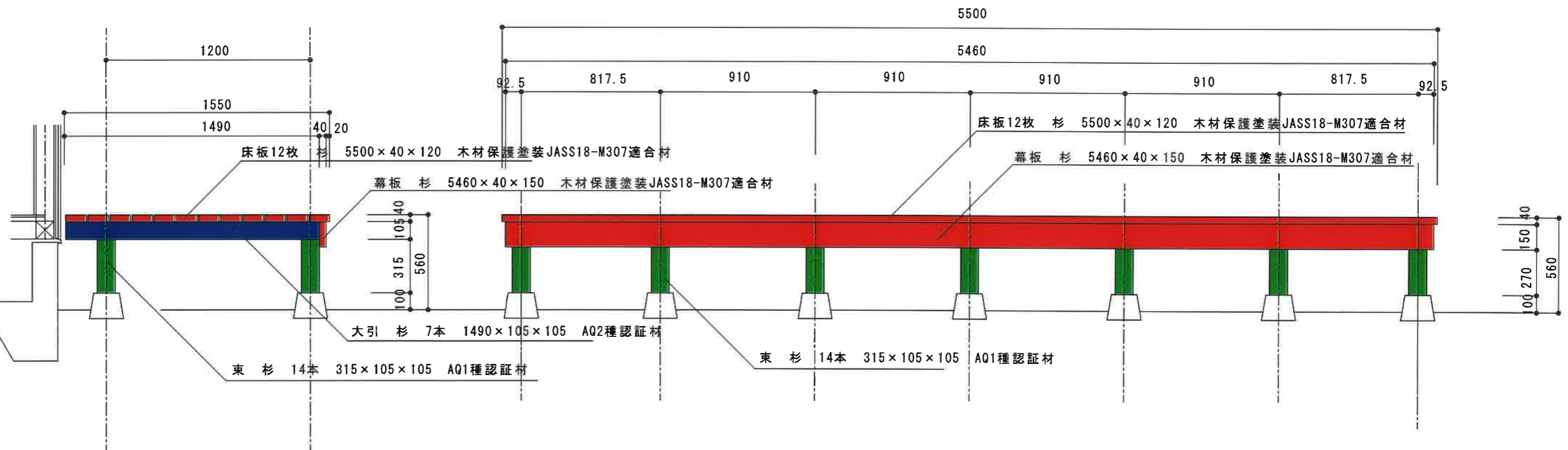
立面図 S=1/25
